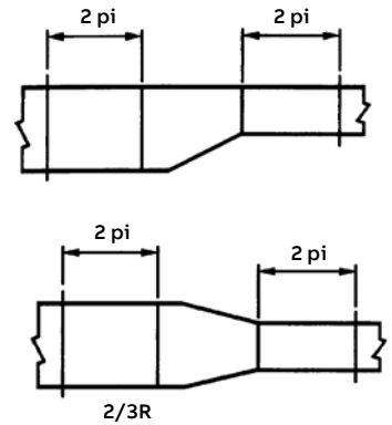
Réducteur horizontal
