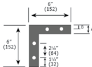
Éclisses 90° verticales
