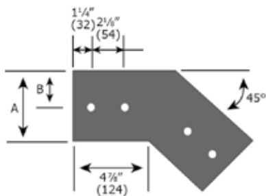
Éclisses 45° horizontales
