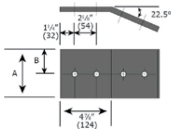
Éclisses 22,5° horizontales
