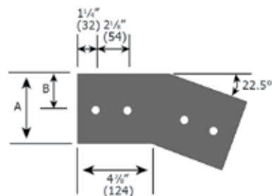
Éclisses 22,5° verticales
