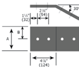
Éclisses 30° horizontales
