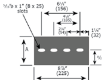
Éclisses d'expansion
