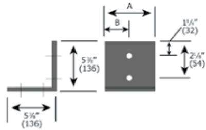
Éclisses 90° horizontales
