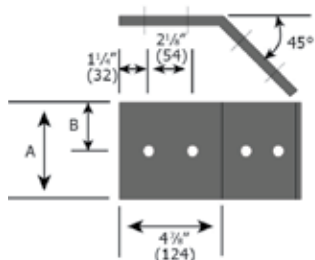
Éclisses 45° verticales
