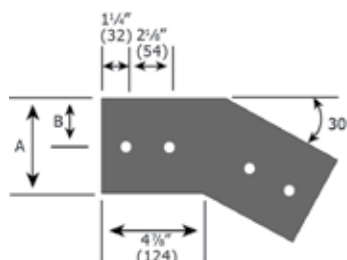
Éclisses 30° verticales
